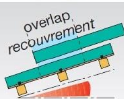
Horní překrytí desek
