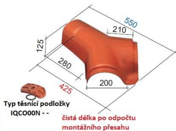
Rozdělovací hřebenáč
