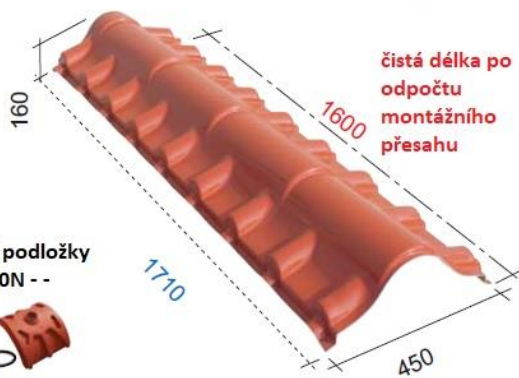
Koncový hřebenáč
